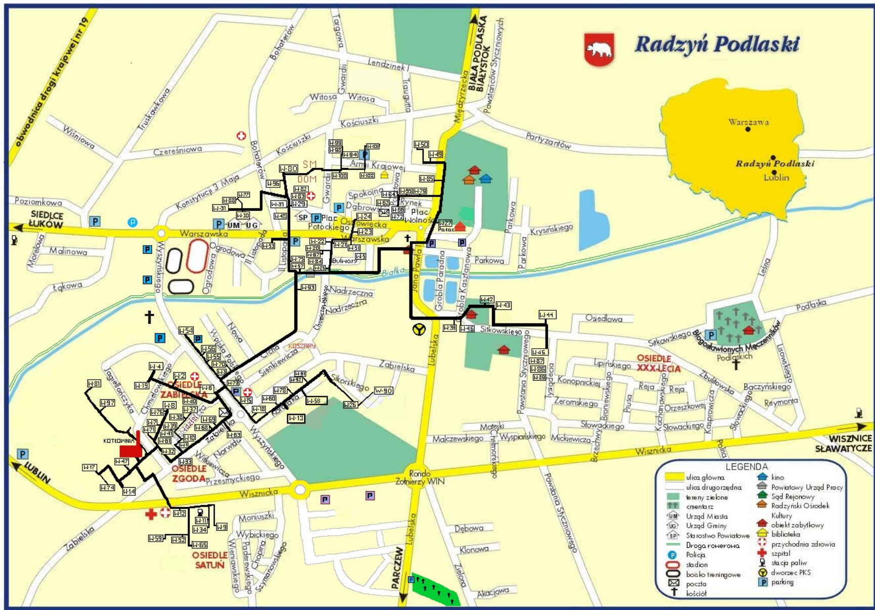
Schemat sieci ciepłowniczej PEC Sp. z o.o. w Radzynie Podlaskim
